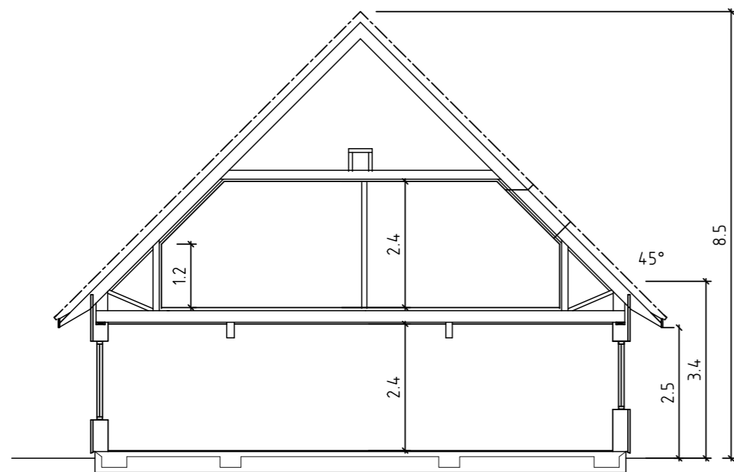
SEKTION A - A
