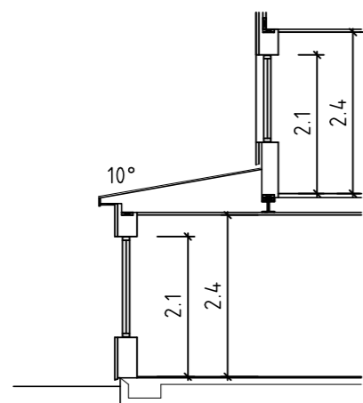
SEKTION B - B
