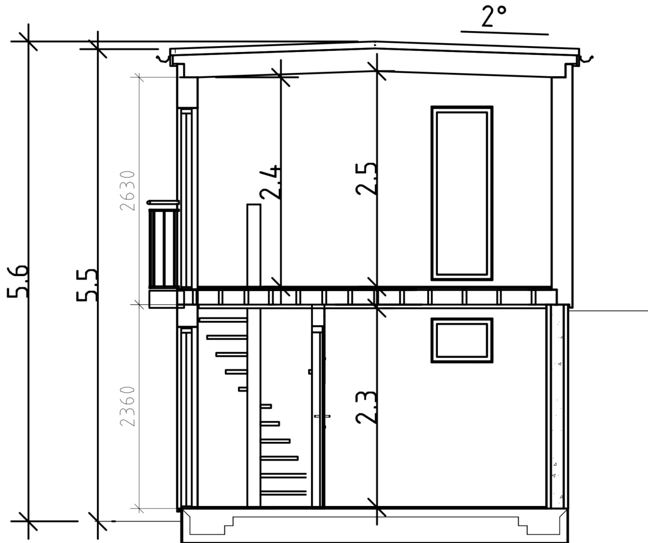
SEKTION A-A
